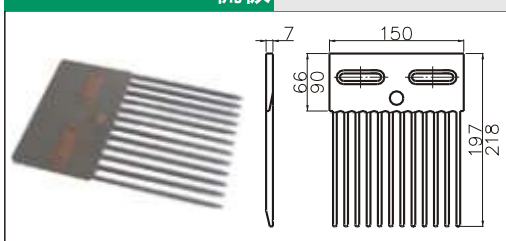
H4707ST12-2梳板
