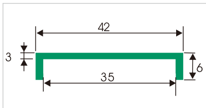
HDS423 盖型垫条
