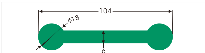
HDS095 哑铃型护栏
