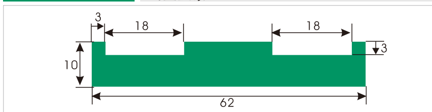
HDS466 山型垫条
