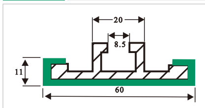
HDS086 大C护栏(带铝合金)
