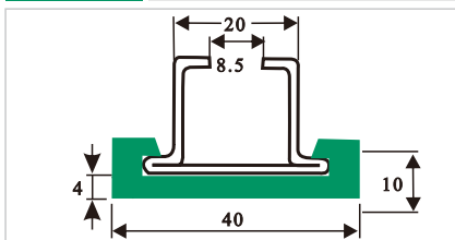
HDS087 盖型护栏(带不锈钢)
