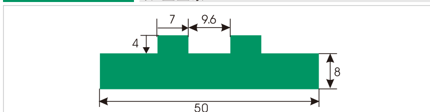
HDS469 双T型垫条
