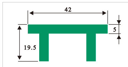
HDS024 TT型垫条
