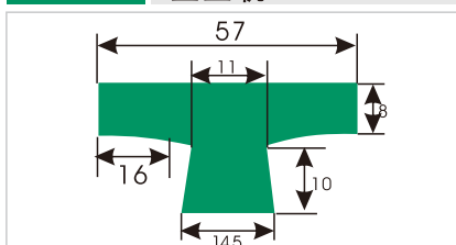
HDS435 T型垫轨
