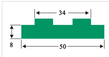
HDS066 T型垫条
