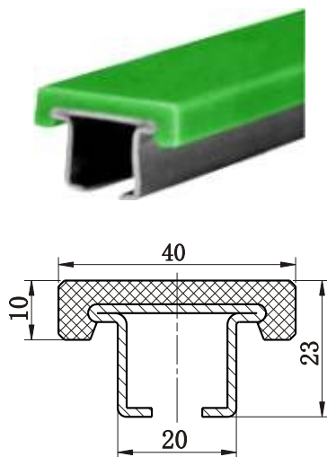
平型垫条
