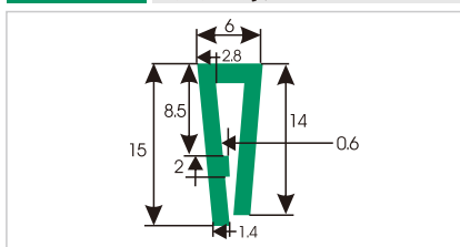
HDS475 U型垫条
