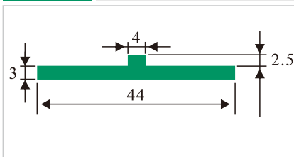
HDS050 T型垫条
