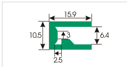
HDS408 U型条
