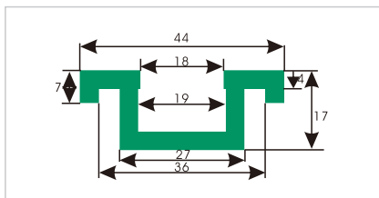
HDS409 TU型垫条
