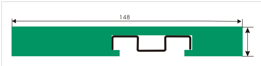
HDS100 高栏-B(单边、带工型钢)
