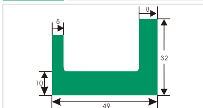
HDS094 U型垫条
