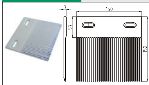
H4803T32梳板
