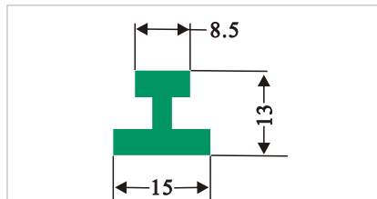
HDS073 工型垫条
