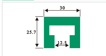
HDS027 链托槽 12B
