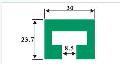
HDS028 链托槽 8B
