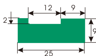
HDS455 U型垫条
