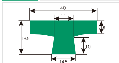
HDS433 T型垫轨
