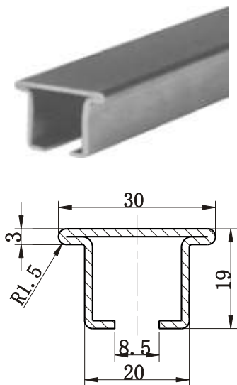
不锈钢垫轨
