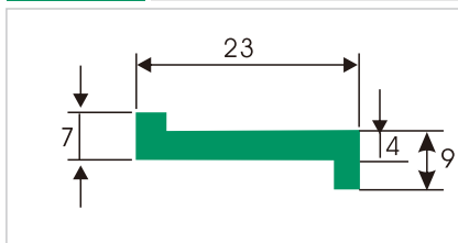
HDS419 Z型垫条
