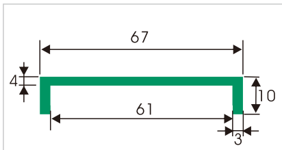
HDS401 盖型垫条
