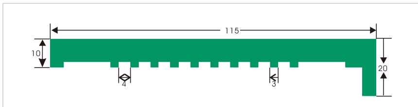
HDS091 L型垫条
