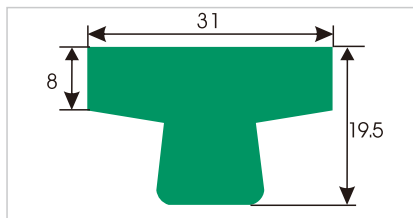
HDS098 T型垫条
