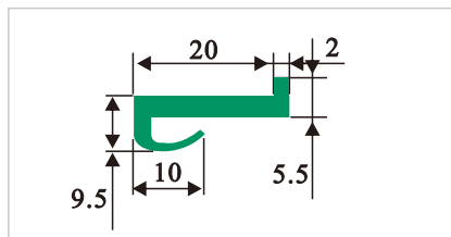
HDS060 K型垫条
