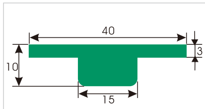
HDS402 T型垫条
