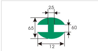
HDS403 工型垫条
