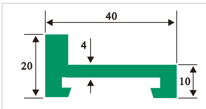
HDS017 L型垫条
