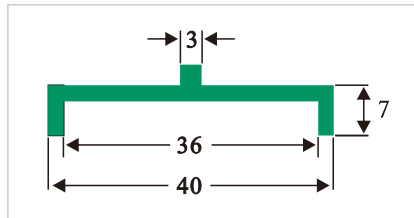
HDS075 宝盖型垫条
