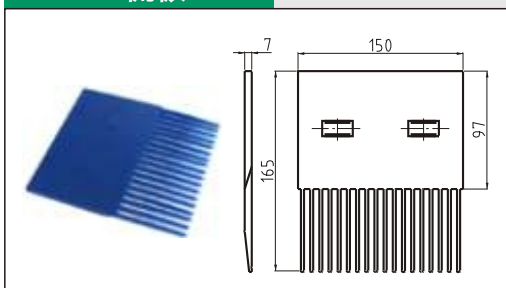
H900梳板
