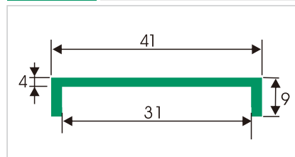
HDS421 盖型垫条
