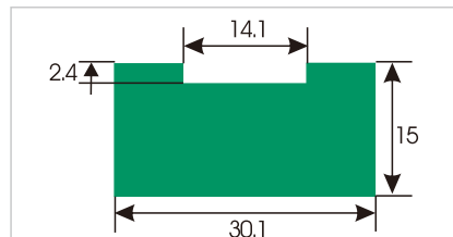
HDS424 U型垫条
