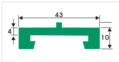
HDS016 宝盖型垫条
