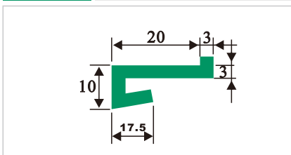
HDS055 K型垫条
