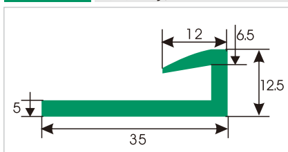
HDS428 K型垫条
