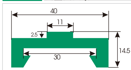
HDS468 宝盖型垫条
