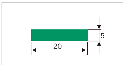
HDS426 平面垫条
