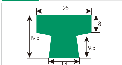
HDS441 T型垫轨
