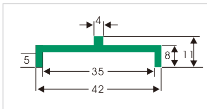
HDS415 宝盖型垫条
