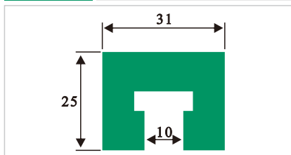
HDS029 链托槽 10B
