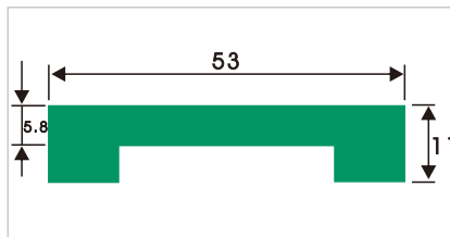
HDS015 盖型垫条
