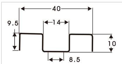
HDS084 工型钢
