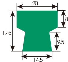
HDS454 T型垫条
