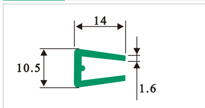
HDS025 小U型垫条
