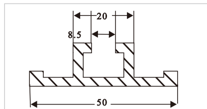
HDS085 铝合金
