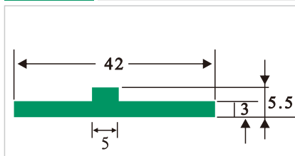
HDS045 T型垫条
