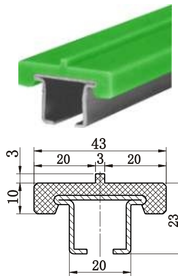
T型垫条
