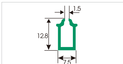
HDS096 U型扣条ABS
