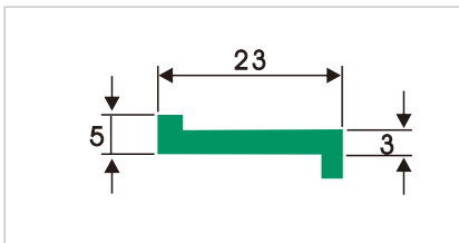
HDS008 Z型垫条
