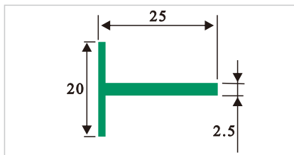
HDS023 T型垫条
