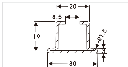
HDS082 平型垫轨(不锈钢)
