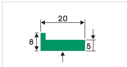
HDS009 L型垫条
