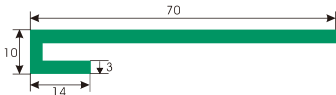
HDS446 K型垫条
