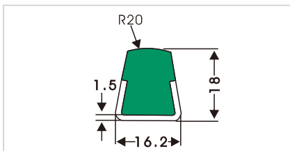
HDS081 D型护栏B(带不锈钢)
