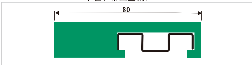
HDS090 中栏(带工型钢)
