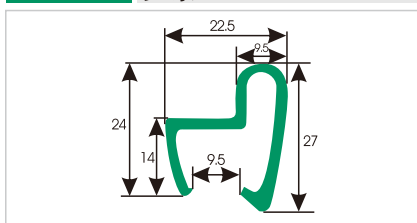
HDS443 扣条
