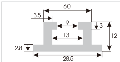
HDS101 铝合金平型垫轨
