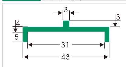
HDS445 宝盖型护栏
