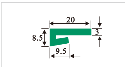
HDS056 K型垫条
