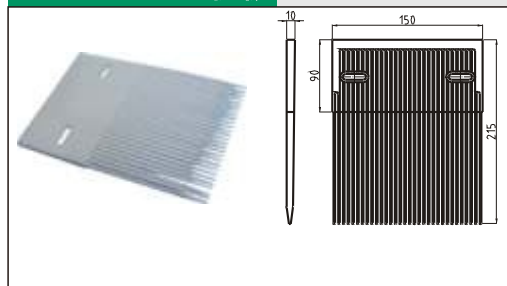
H2037T28梳板
