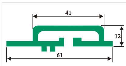
HDS039 大号饰条ABS
