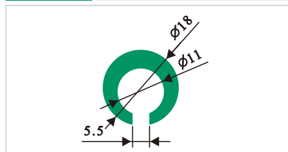
HDS030 套管护栏
