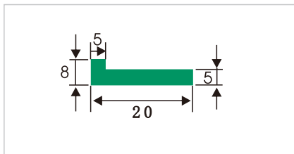
HDS406 L型垫条
