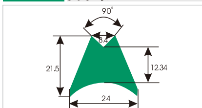
HDS429 支承条
