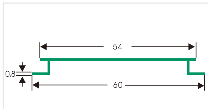
HDS076 宝盖型垫条
