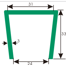
HDS460 U型垫条
