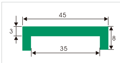
HDS414 盖型垫条
