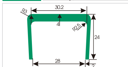
HDS465 U型垫条
