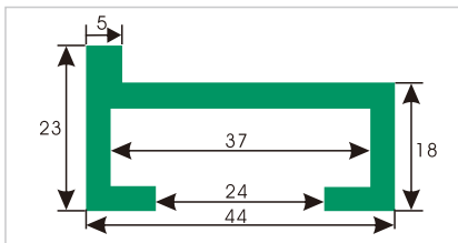
HDS407 低栏B型
