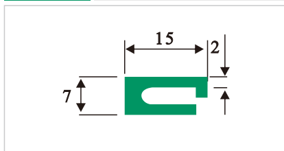
HDS026 G型扣条
