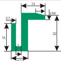
HDS448 Z型垫条
