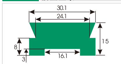
HDS470 槽型垫条
