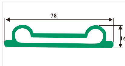
HDS018 中空护栏
