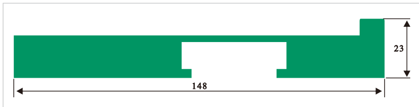
HDS033 高栏-B(单边)
