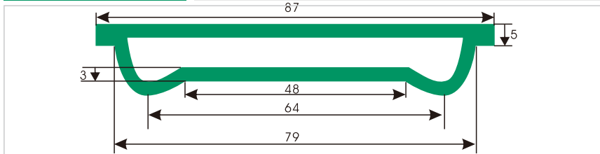
HDS416 中空护栏
