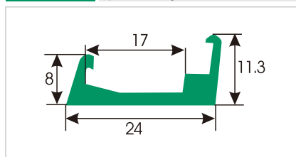
HDS442 槽型垫条
