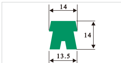
HDS020 平顶护栏B款
