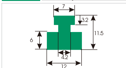
HDS444 工型垫条
