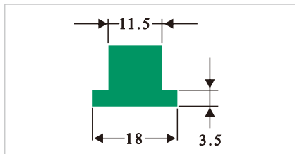
HDS068 T型垫条
