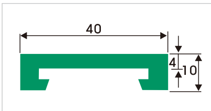
HDS014 盖型垫条
