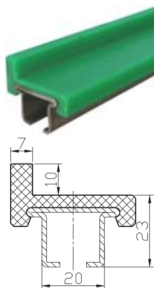
L盖型垫条
