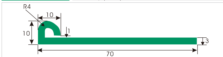
HDS464 K型垫条(圆顶)
