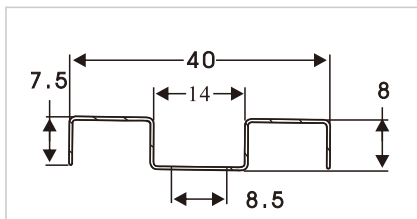
HDS083 工型钢
