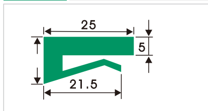
HDS012 K型垫条
