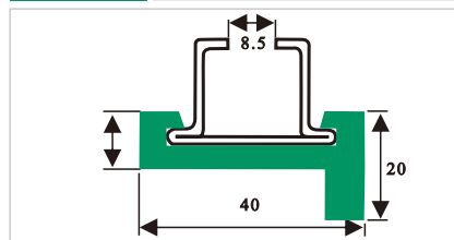
HDS088 L型护栏(带不锈钢)
