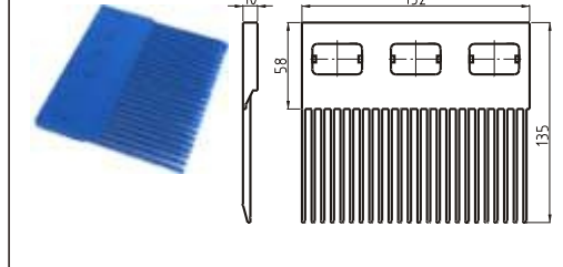
H4803T32梳板
