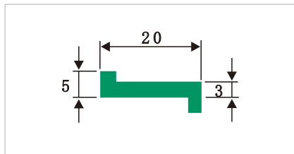
HDS007 Z型垫条
