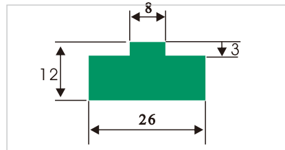
HDS417 T型垫条
