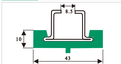
HDS089 宝盖型护栏(带不锈钢)
