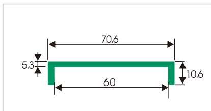
HDS412 盖型垫条
