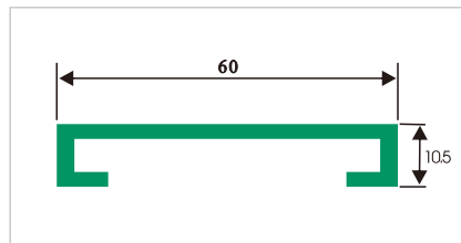
HDS092 大C护栏(自配)
