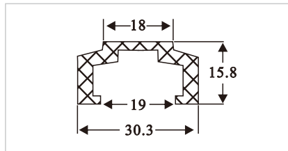
HDS067 套铝合金护栏
