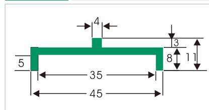
HDS418 宝盖型垫条
