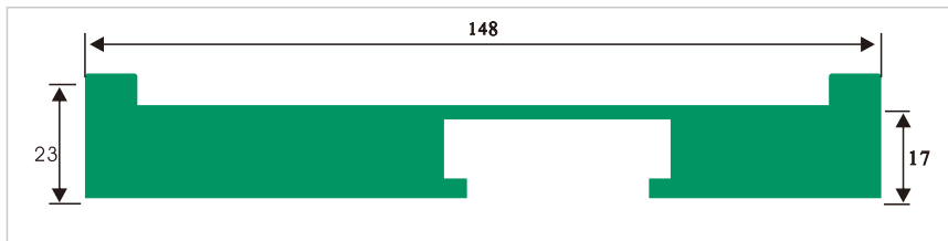
HDS032 高栏-A(双边)
