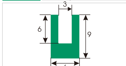
HDS467 U型垫条
