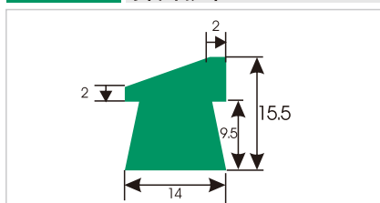
HDS474 斜面护栏
