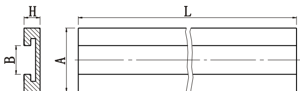
HT882-K750 — 链的宽度 — 链的型号 — 单列直导轨
