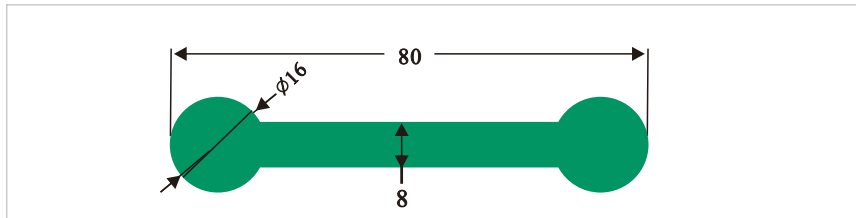
HDS74 哑铃型护栏
