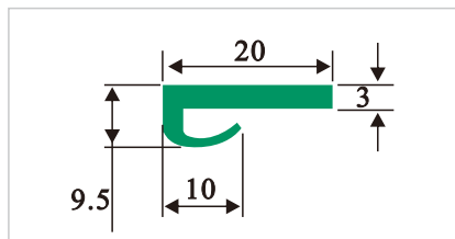
HDS061 K型垫条
