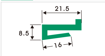
HDS011 K型垫条
