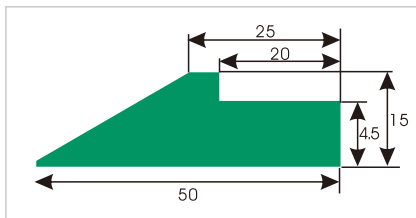
HDS422 箭型垫条
