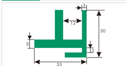
HDS431 网链卡条
