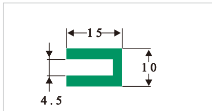
HDS071 U型垫条
