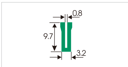
HDS097 U型压条ABS
