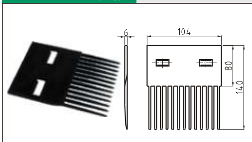
H5937T15梳板
