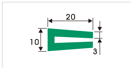
HDS013 U型垫条
