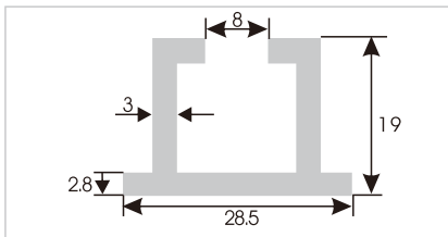
HDS102 铝合金平型垫轨
