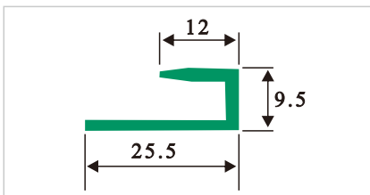
HDS040 中号饰条ABS
