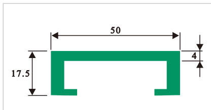
HDS031 低栏
