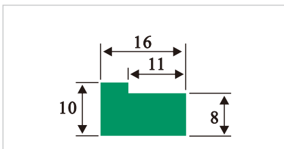
HDS036 L型垫条
