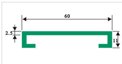
HDS022 大C护栏
