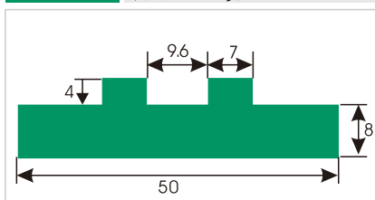
HDS457 双T型垫条
