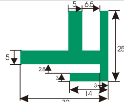
HDS451 F型垫条
