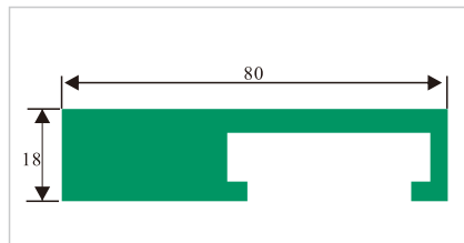
HDS034 中栏
