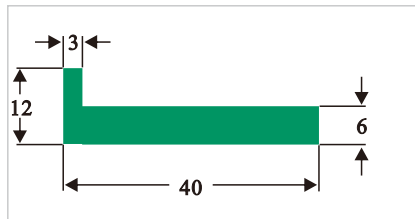
HDS072 L型垫条
