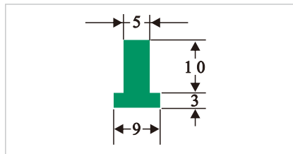
HDS069 T型垫条
