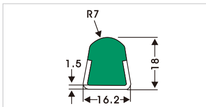
HDS080 D型护栏A(带不锈钢)
