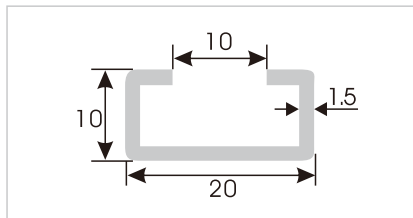
HDS103 C型钢
