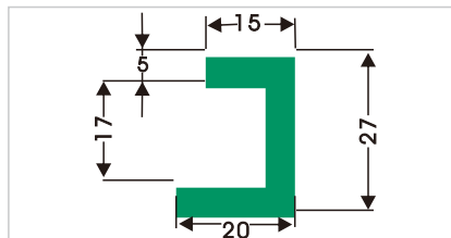
HDS078 中空护栏
