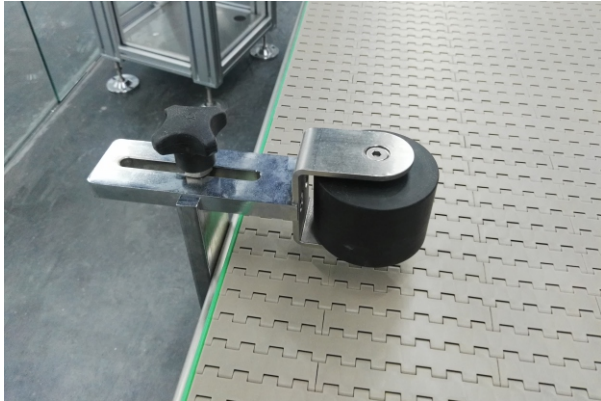
▶ 转向小机构
