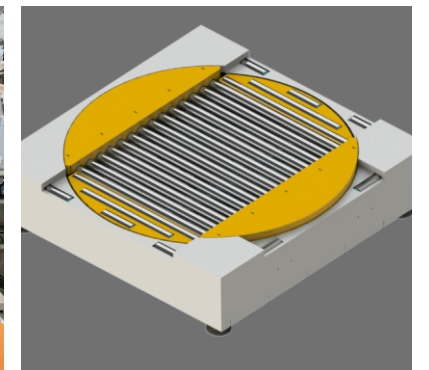
▶ 重型转向机
