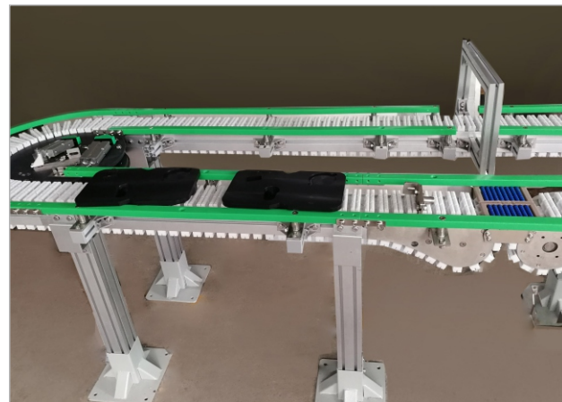
带滚珠柔性链
